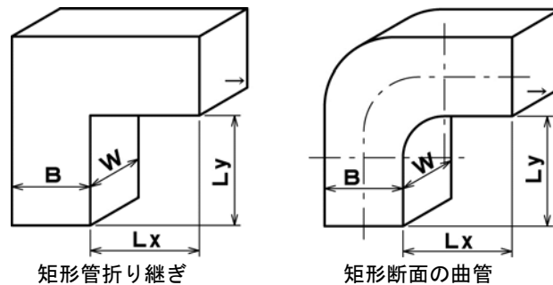
図・1 矩形管折り曲げダクトの形状例
