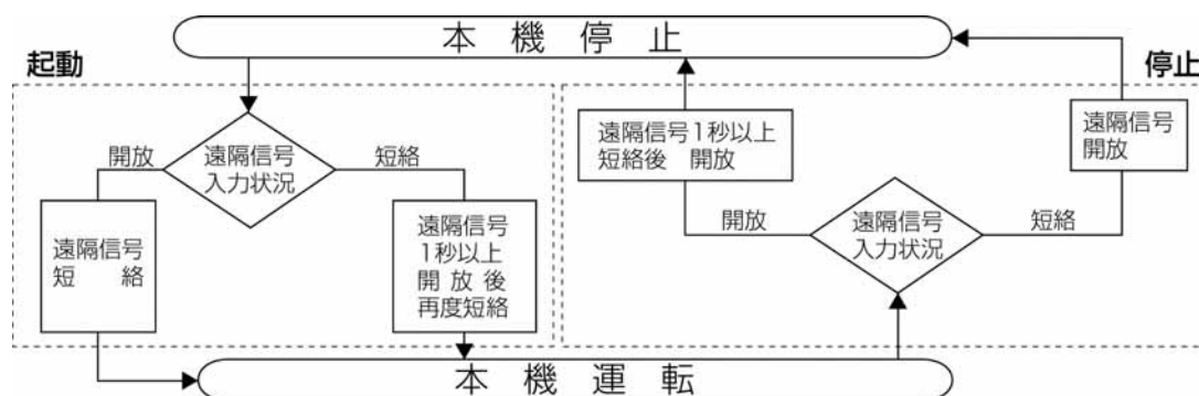
遠隔操作動作フローチャート
