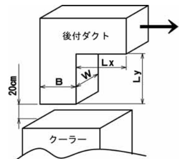
図・2 Lx および Ly の長さが2mを超える場合のダクト取付方法
