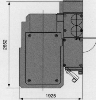
サーマルガード仕様 フロア図
