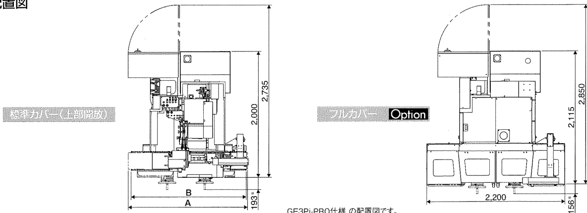
GE3Pi-PRO仕様の配置図です。 *はGE3Pi-PROの前面ハンドル付属特有の寸法です。
