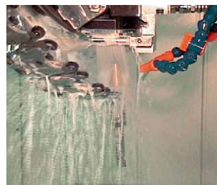
工具テーパ部を洗浄する様子
