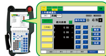
機械操作画面
