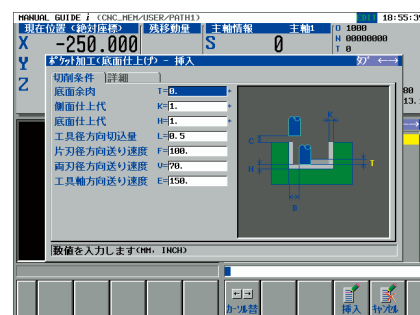
加工サイクル入力画面
