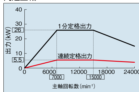
高速主軸
