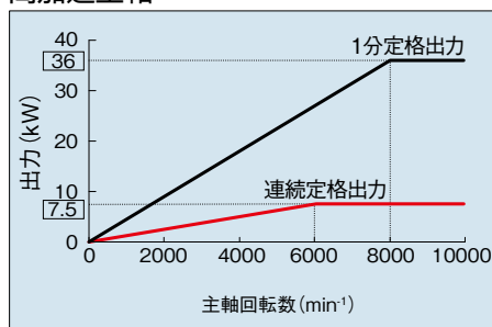
高加速主軸
