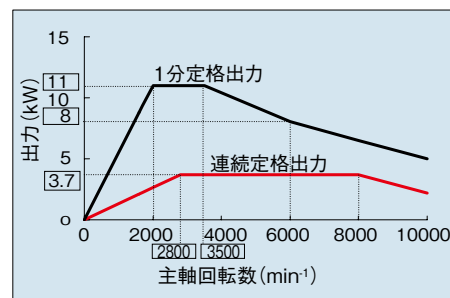
標準主軸
