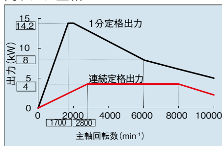
高トルク主軸
