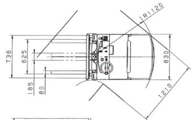
りとる RUNNER FBT5
