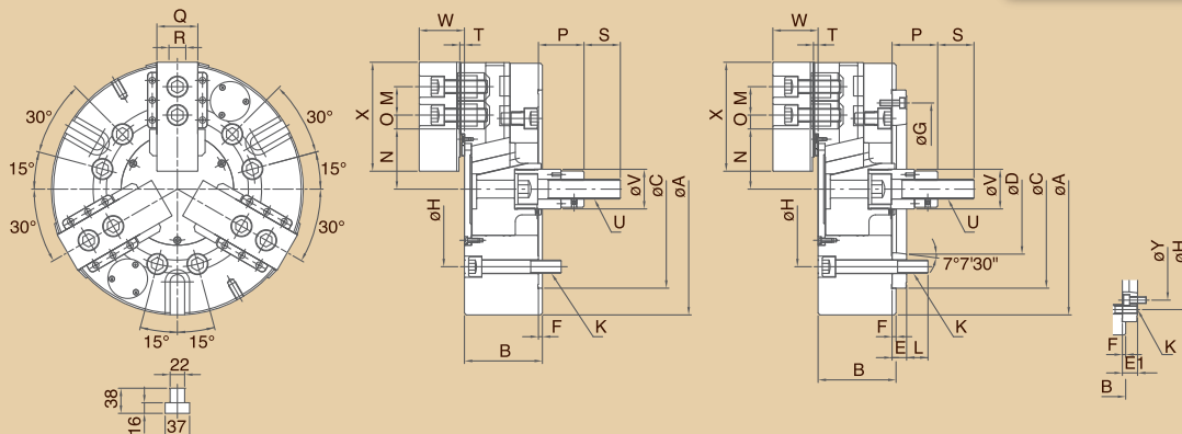
寸法図
