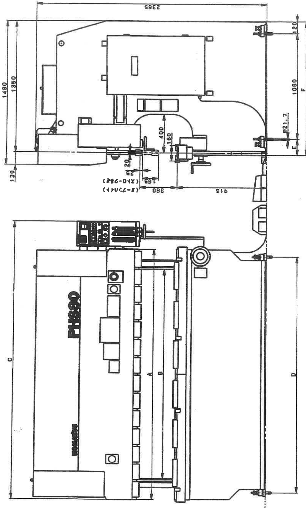
機械の寸法 (PHS80 × 200, 255, 310-21)
