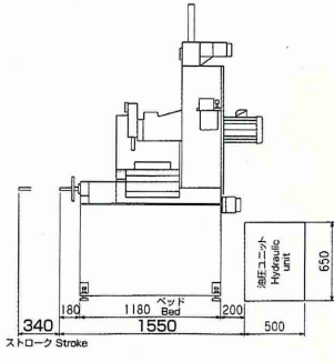
加工範囲 GRINDING RANGE
