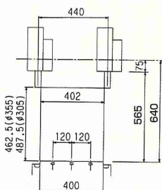
加工範囲 GRINDING RANGE
