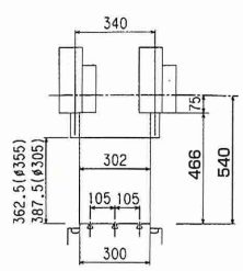
加工範囲 GRINDING RANGE
