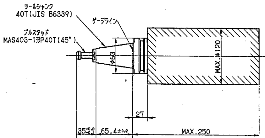
図1. 1 工具最大寸法 (40T JIS B6339)
